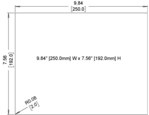
Cutout Dimensions
