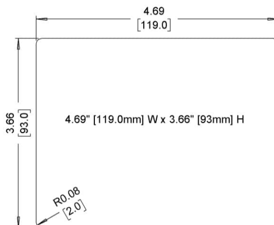
Cutout Dimensions
